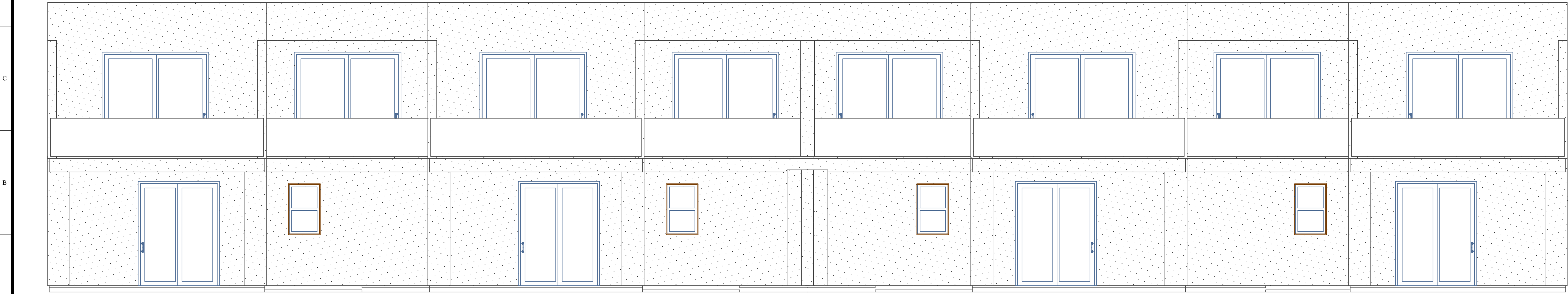
A1 Back Elevation SCALE: 1/4" = 1'-0"
